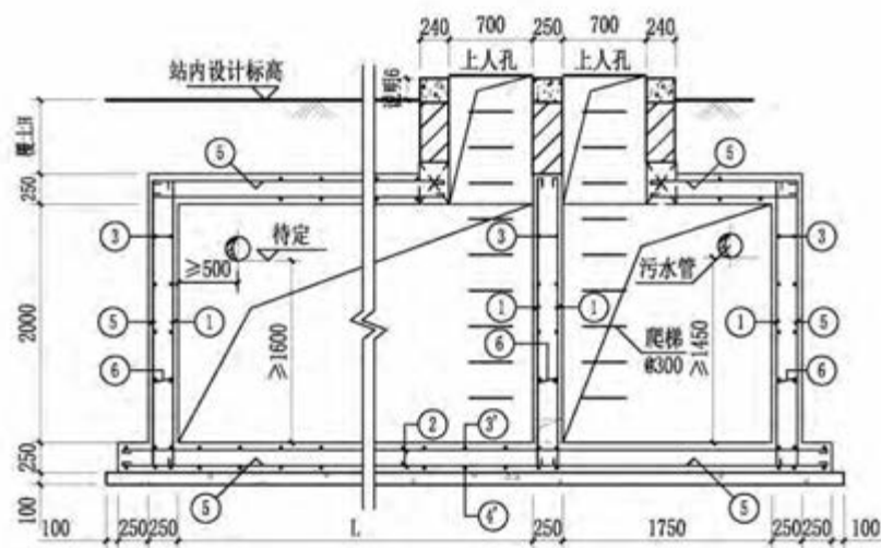
2-2剖面图 1:40
