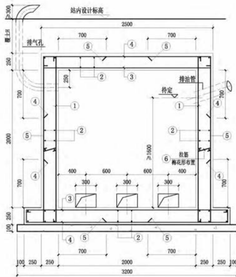
1-1剖面图 1:20
