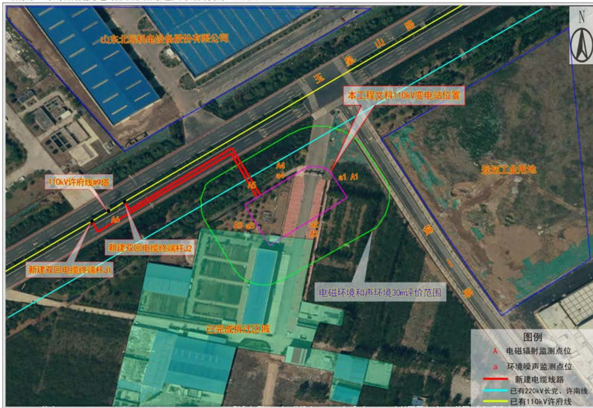
附图4 环评阶段变电站及线路周边关系影像图 比例尺1:2000
