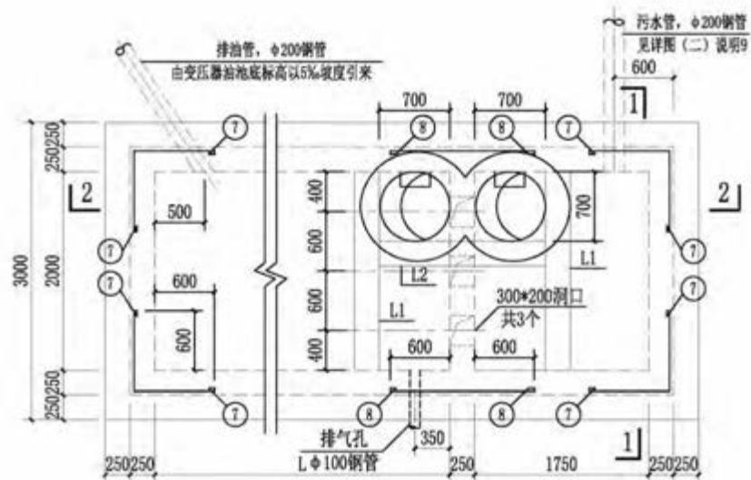
事故储油池平面图 1:40
